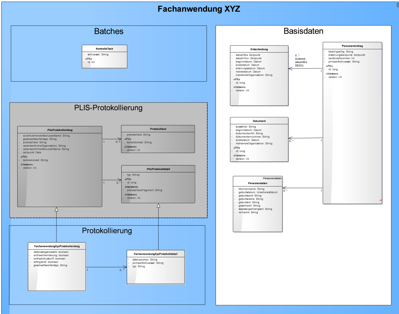
Abbildung 8. Logisches Datenmodell
